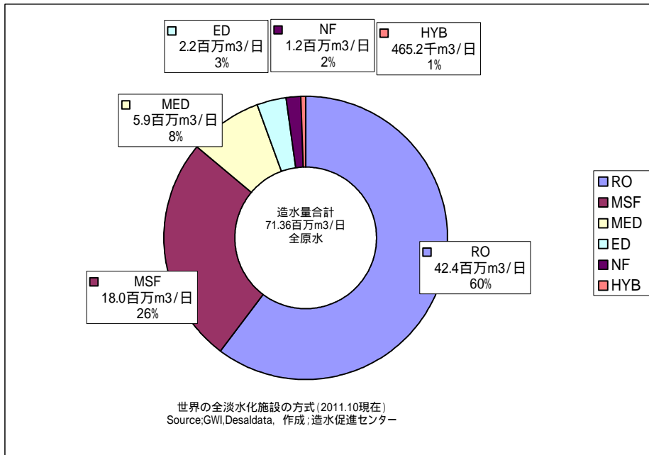
図5 世界の淡水化施設の方式別割合 (海水以外も含む、運転開始 2011 年まで)
