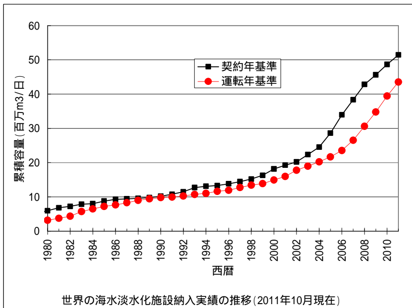
図6 世界の海水淡水化施設納入実績の推移 (海水のみ、運転開始 2011 年まで)
